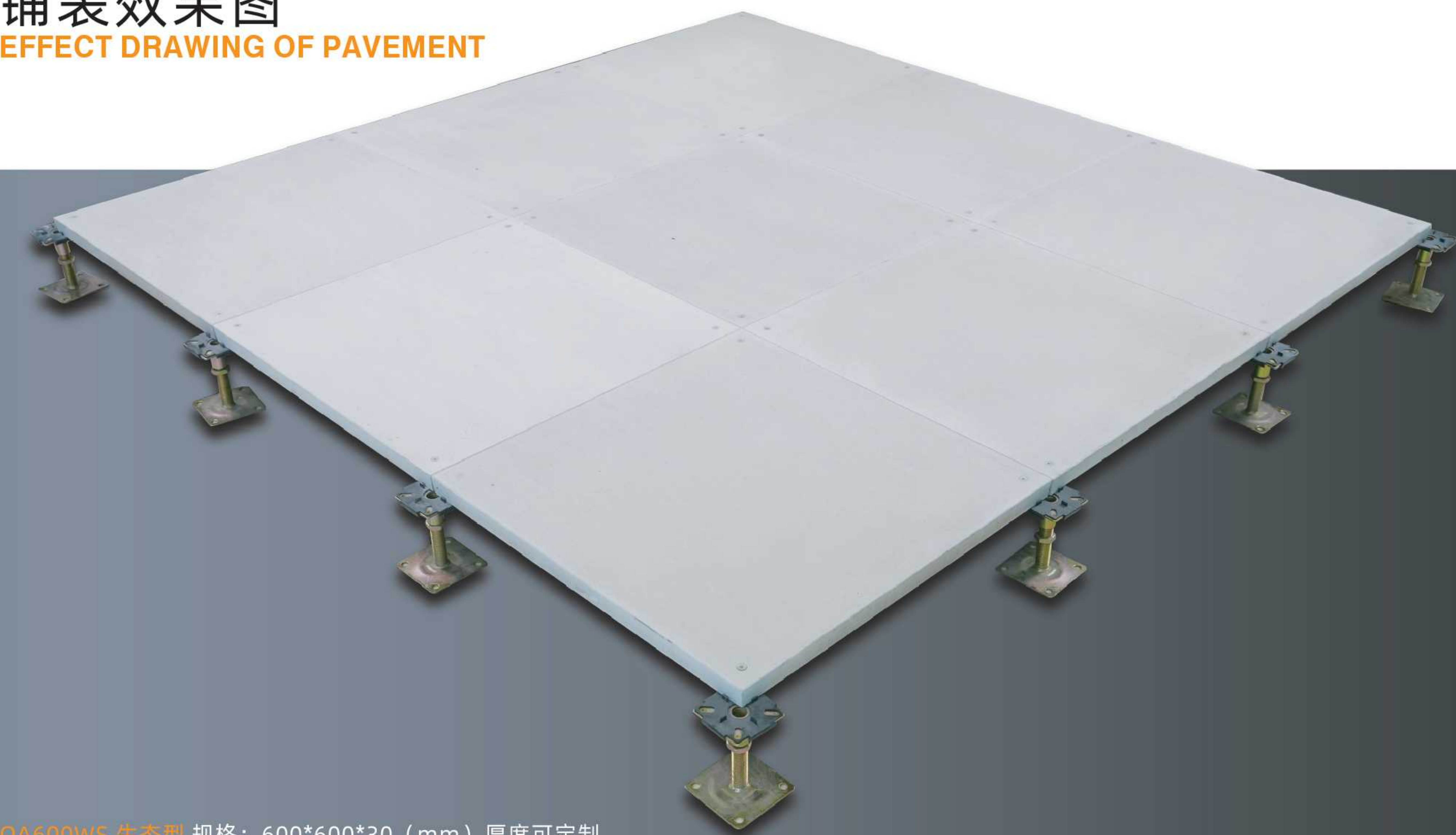
OA600WS 生态型 规格：600*600*30（mm）厚度可定制 OA500WS 生态型 规格：500*500*30（mm）厚度可定制
