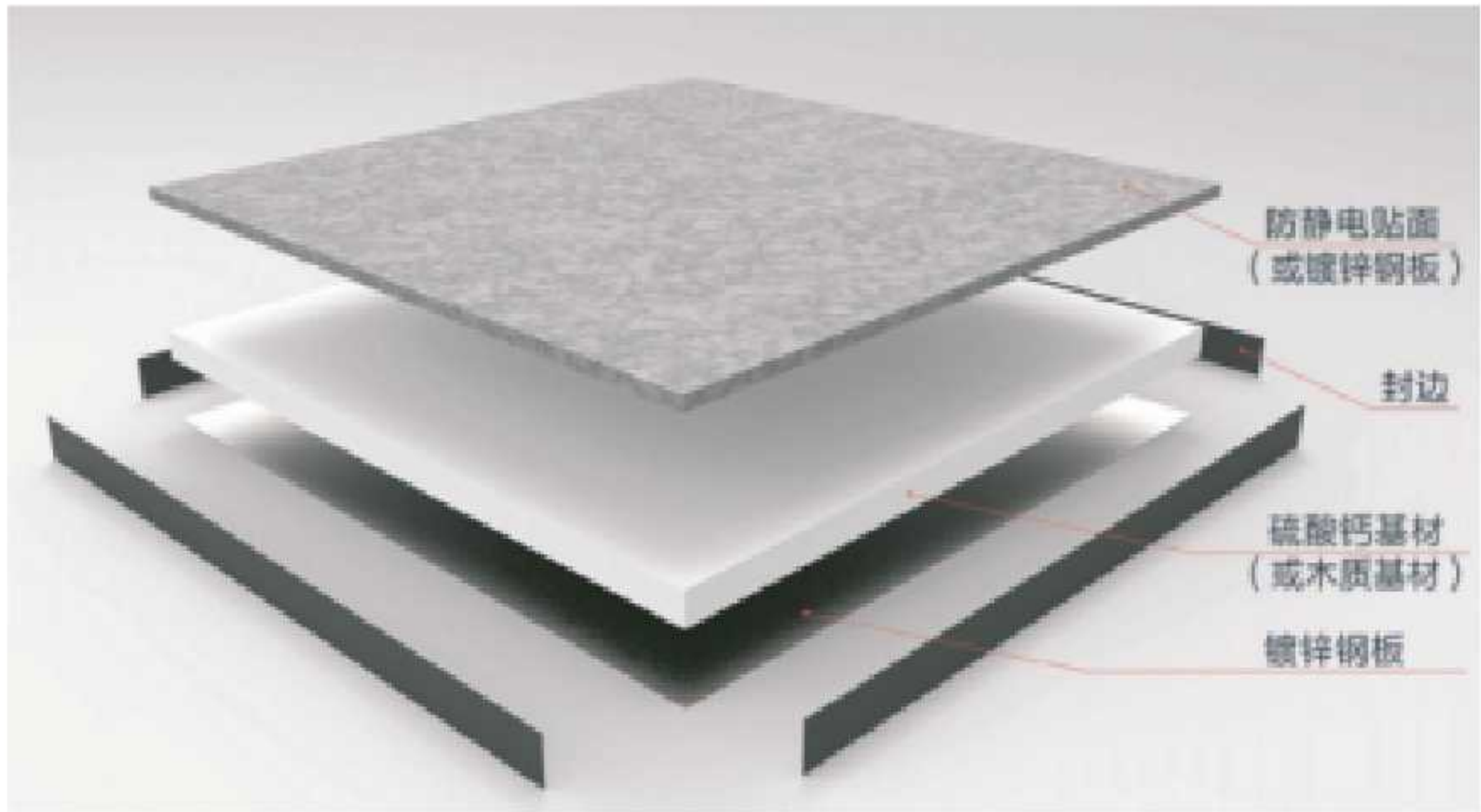
硫酸钙防静电活动地板组成结构示意图
