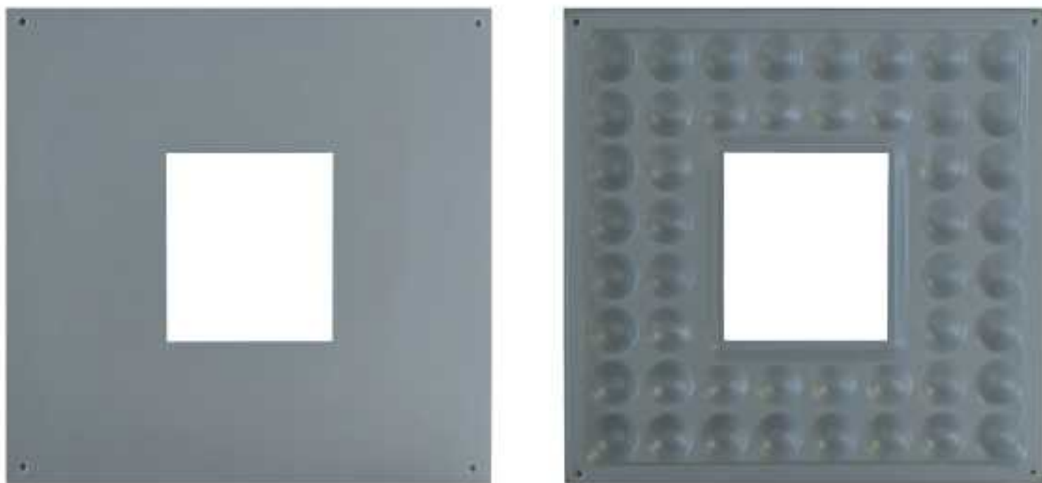
OA600 钢质网络模开孔地板 开孔尺寸 *Hole Size 230*220mm 配套地插座面板尺寸 250*220mm
