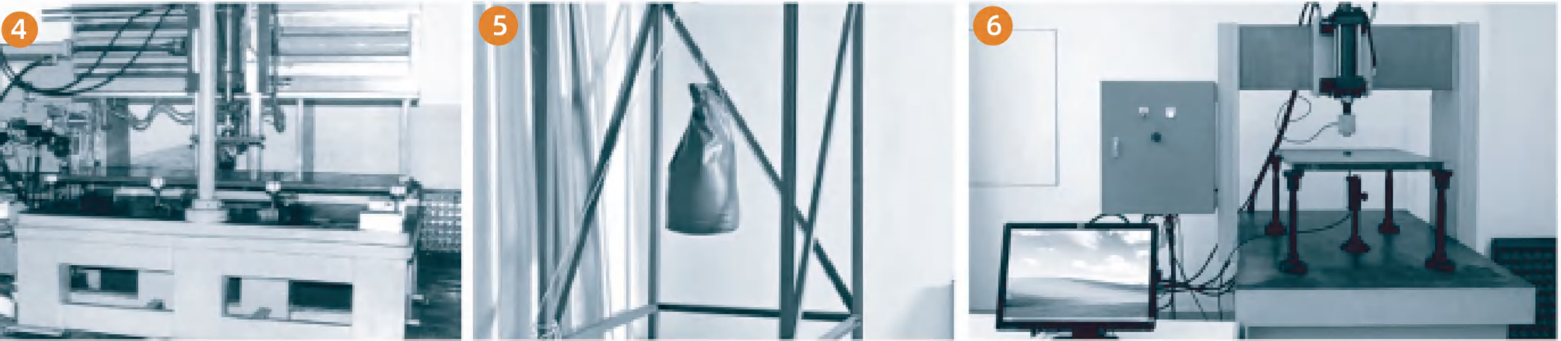
④ 滚动荷载测试/Rolling load test ⑤ 沙袋冲击测试/Sandbag impact test ⑥ 集中荷载测试/Concentrated load
