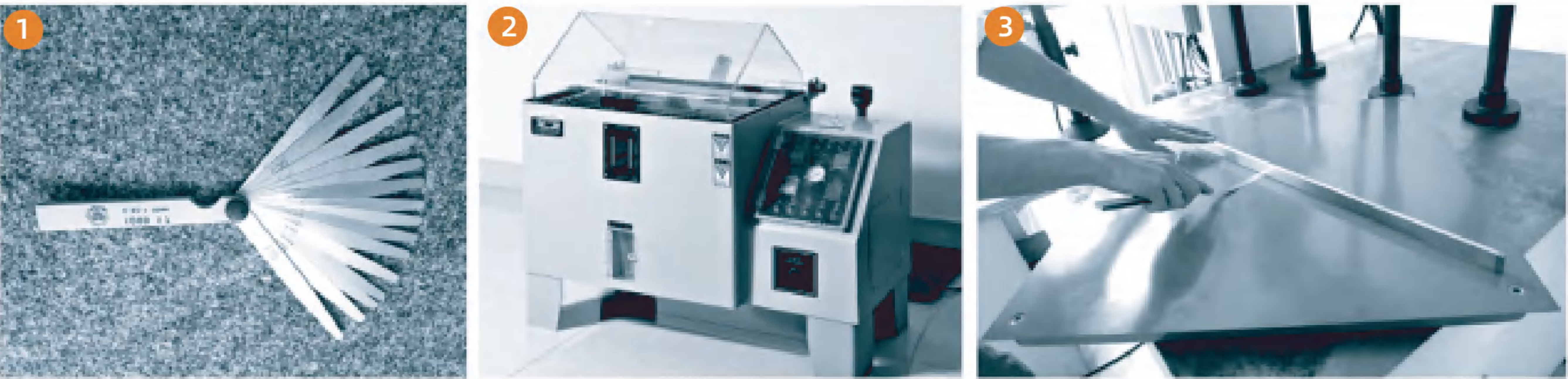
① 检测器具 塞尺/inspection tool ② 盐雾测试/Salt fog test ③ 平整度测试/Flatness test
